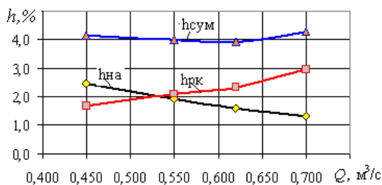
Рис. 6 – Потери энергии в направляющем аппарате и рабочем колесе
