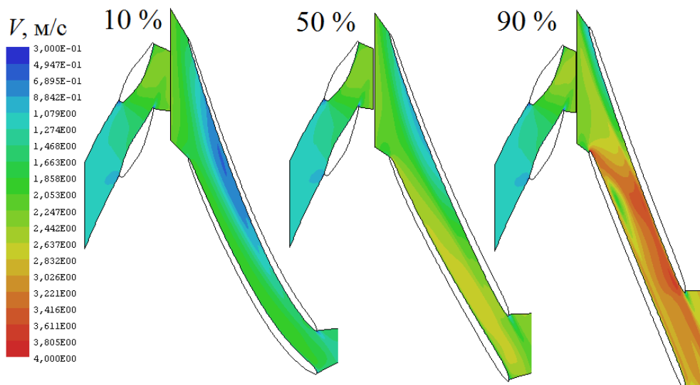
Рис. 4 – Распределение скорости потока V в области НА и РК в тангенциальном сечении при оптимальном значении расхода Q_1' = 620 л/с.
