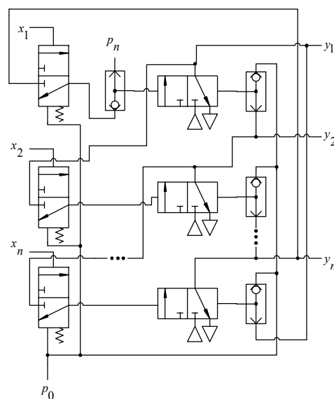
Рис. 2 – Схема командоаппарата
