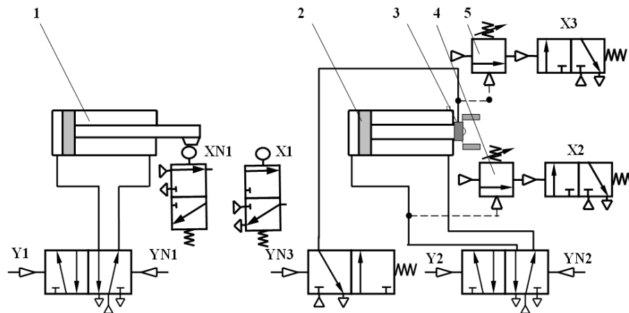
Рис. 1 – Приклад схеми модуля пневматичного маніпулятора:
